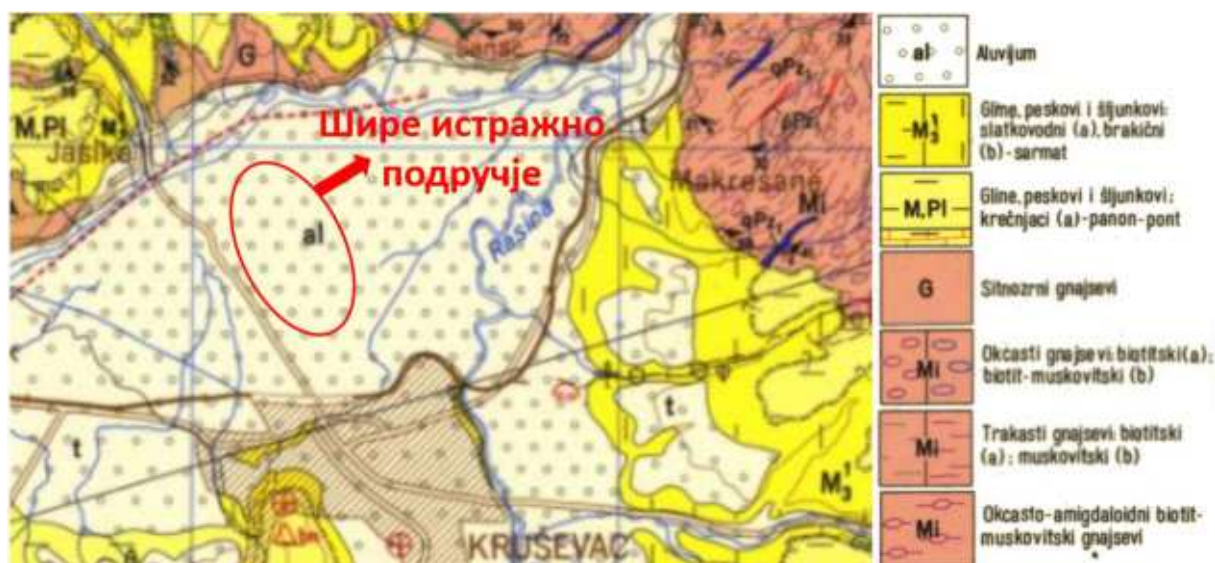
Слика бр. 10: Геолошка грађа ширег истражног подручја, исечак из Основне геолошке карте, лист Параћин К 34-7, размере 1:100.000, са легендом
